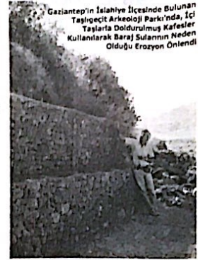
Gaziantep'in İslahiye İlçesinde Bulunan Taşlıçiftlik Arkeoloji Parkı'nda, İçine Taşlarla Doldurulmuş Çelik Kafesler Kullanılarak Baraj Sularının Neden Olduğu Erozyon Önlenildi
